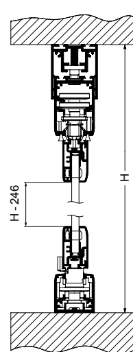
Superior con expansor Inferior sobrepuesto
